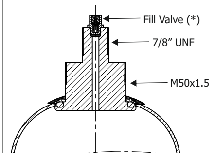
Type : MU7/8
