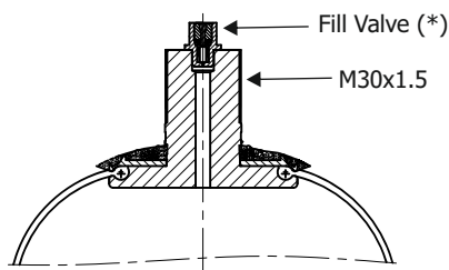
Type : M30
