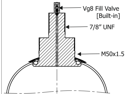
Type : MU7/8V
