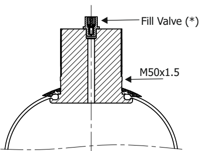
Type : M50
