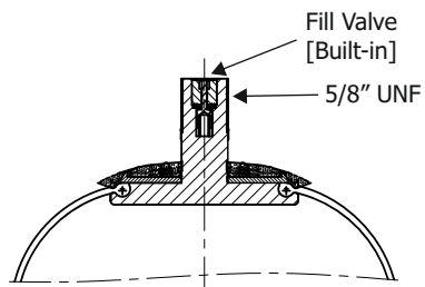
Type : U5/8
