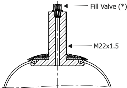
Type : M22L
