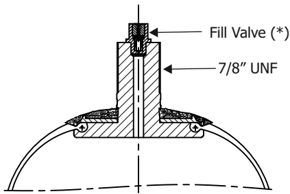
Type : U7/8
